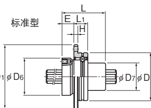
LTR10A型
