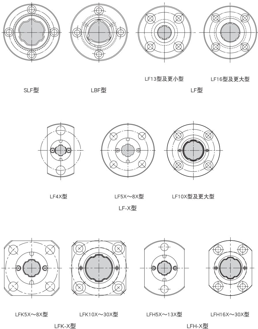
图2 法兰安装孔的位置
