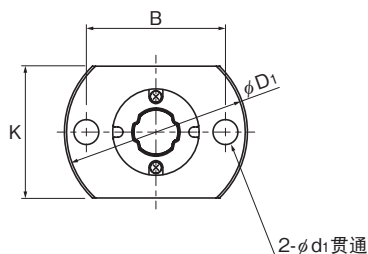
LFH5X~LFH13X
