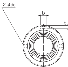
LT13型及更小型
