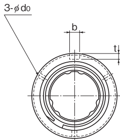
LT16型及更大型
