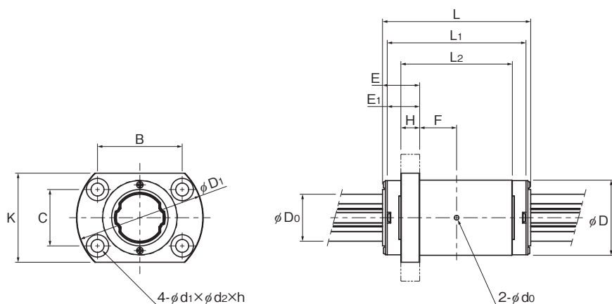
LFH16X~LFH30X
