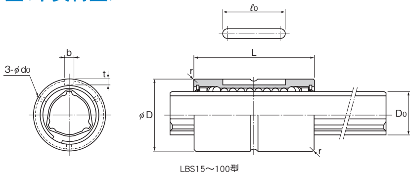
LBS15~100型
